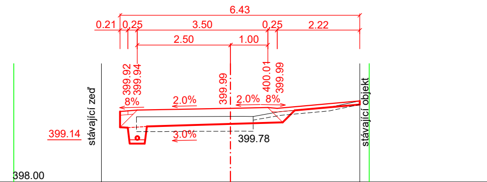
ŘEZ č. 7 - km 0.060 00
