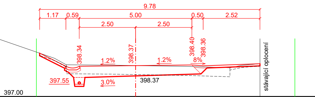
ŘEZ č. 1 - km 0.010 00
