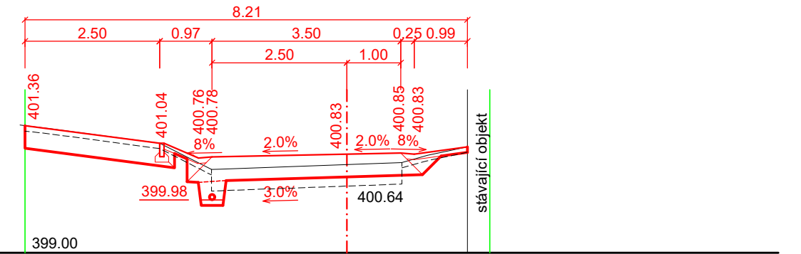
ŘEZ č. 9 - km 0.080 00
