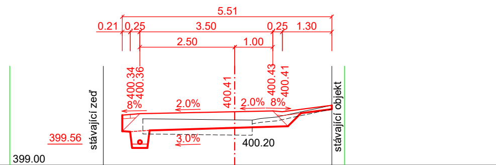
ŘEZ č. 8 - km 0.070 00
