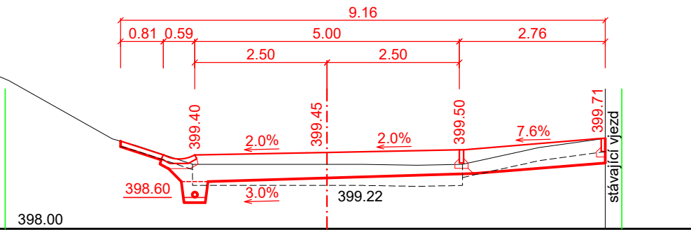
ŘEZ č. 5 - km 0.046 43
