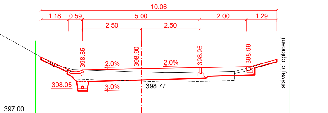
ŘEZ č. 3 - km 0.030 00
