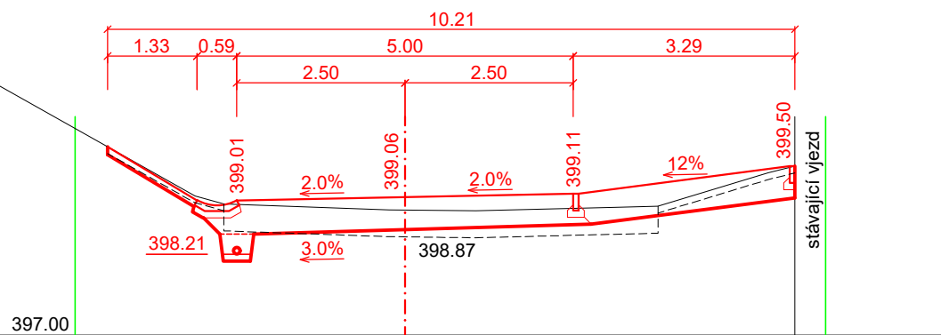
ŘEZ č. 4 - km 0.035 42
