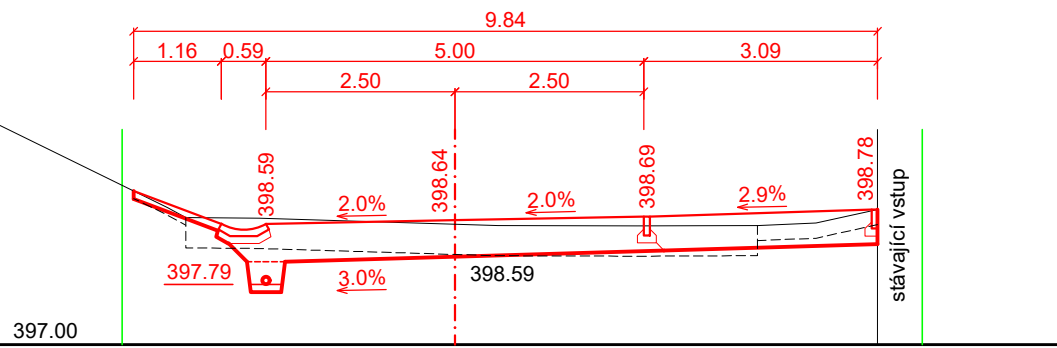
ŘEZ č. 2 - km 0.020 49
