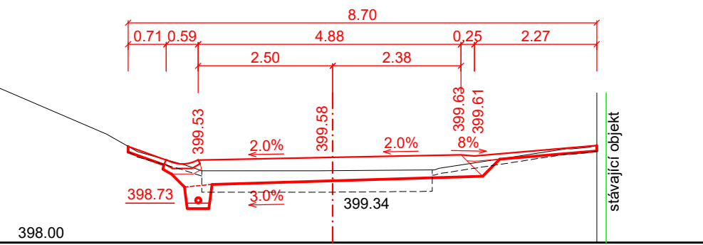
ŘEZ č. 6 - km 0.050 00
