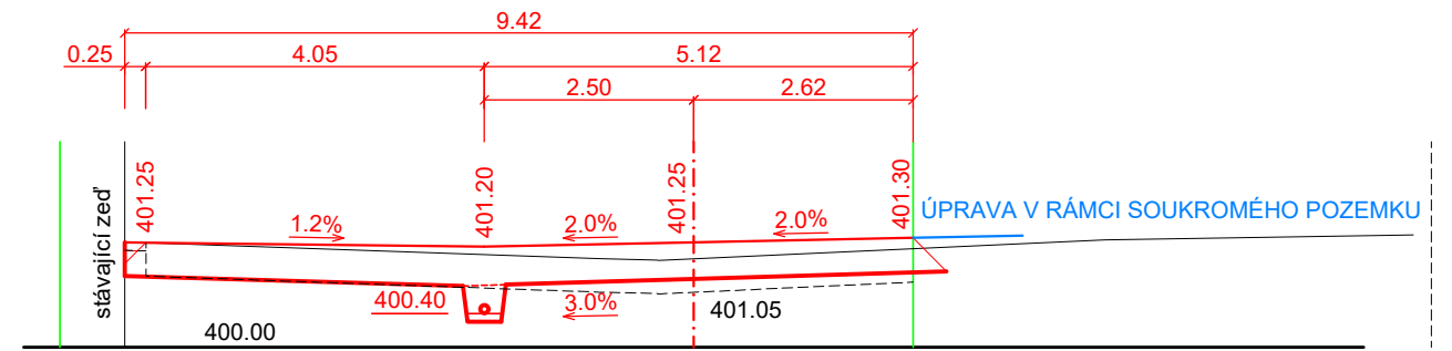
ŘEZ č. 10 - km 0.090 00
